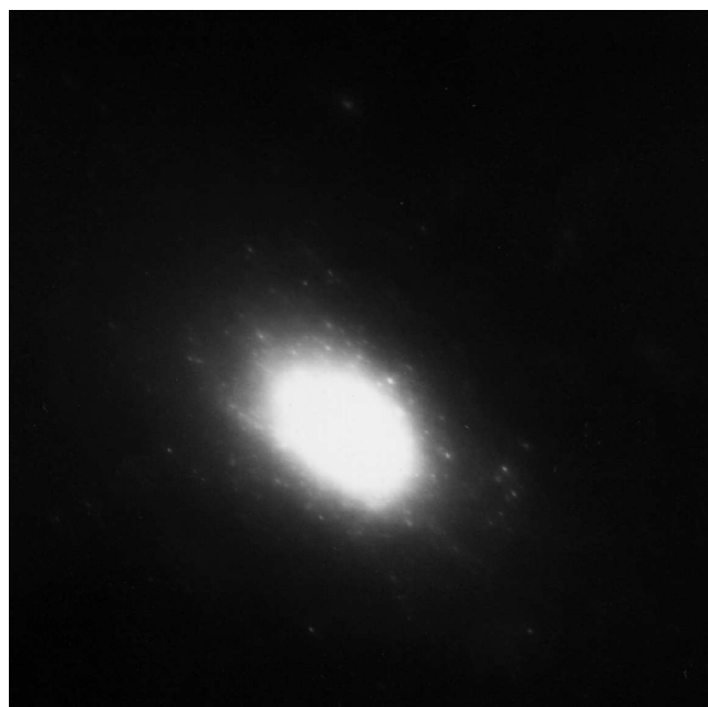
Andrômeda. Família de hadrons detectada na câmara n. 14 da CBJ, a 11 comprimentos de radiação de Pb. A câmara era constituída por 12 cm de Pb intercalados com 10 camadas de filmes de raios-X e placas de emulsão nuclear. A energia do evento foi estimada em 20000 TeV.
